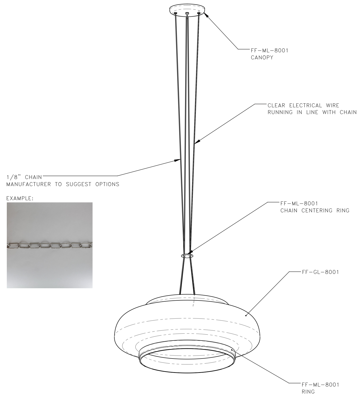
1 LT-8002 PENDANT LIGHT 1:8 ISO FRONT
