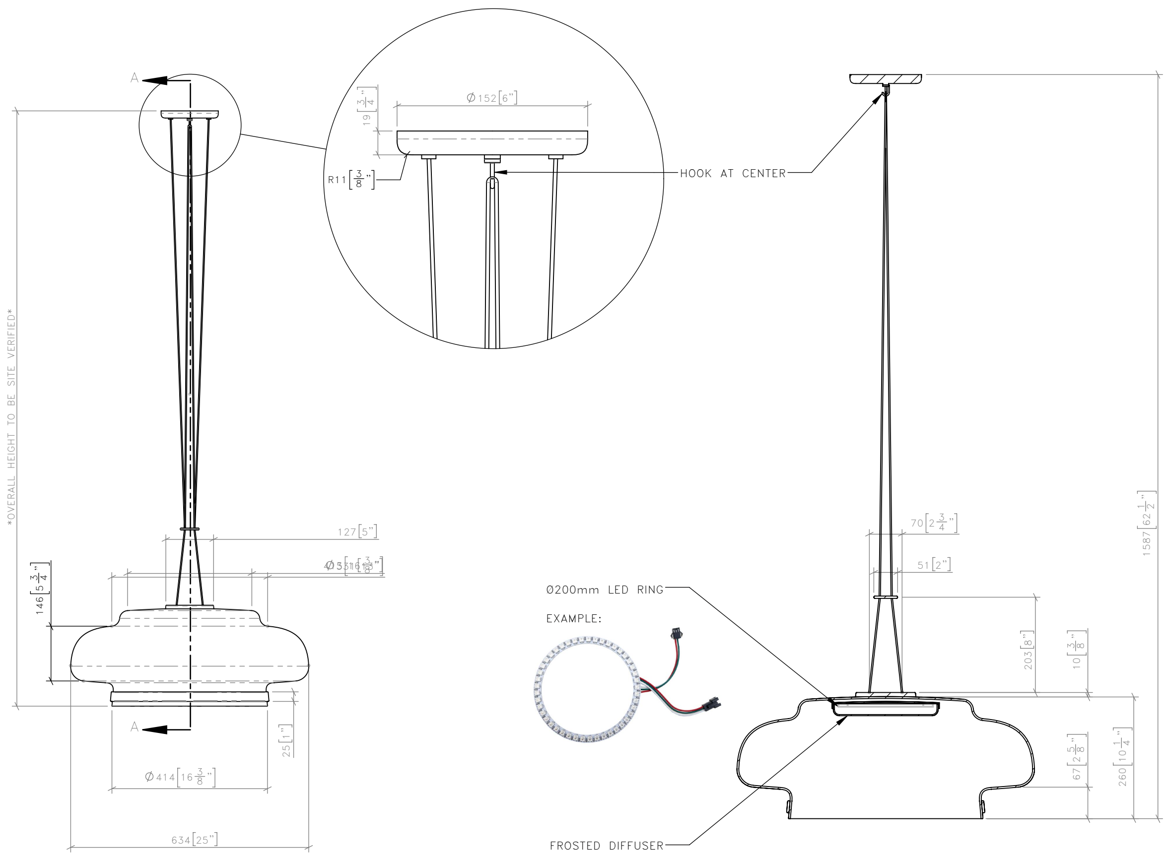
3 LT-8002 PENDANT LIGHT SECTION A-A 1:10
