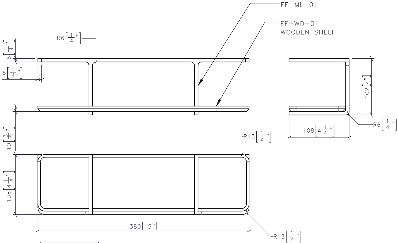
11 CG-310 MINIBAR 1:16 CUSTOM DOOR SHELF
