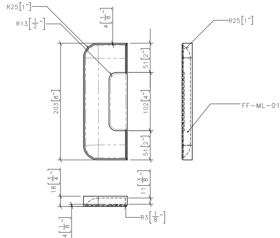
10 CG-310 MINIBAR 1:16 CUSTOM DOOR PULL
