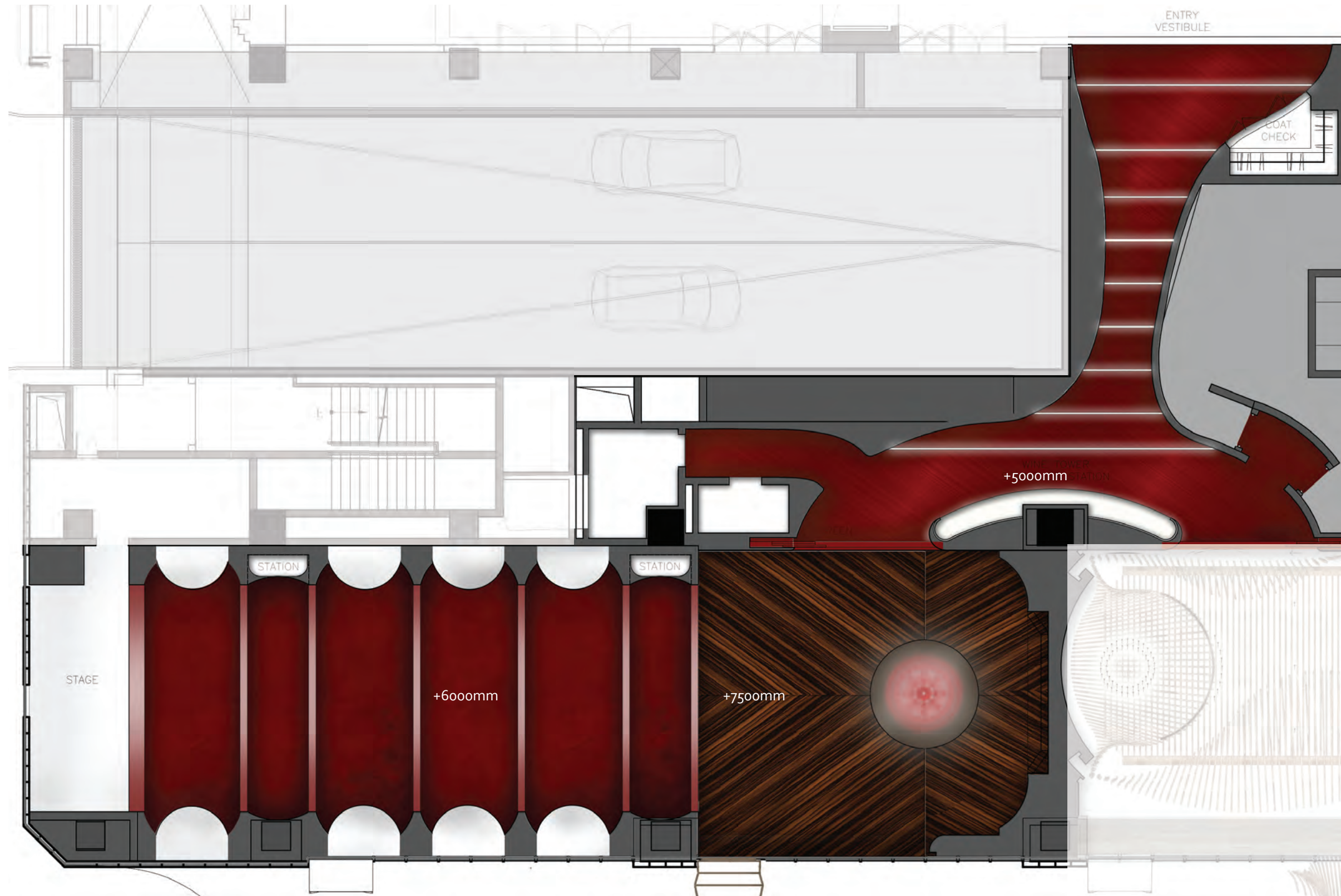
QING BAR RCP - "QING" 酒吧 天花图
