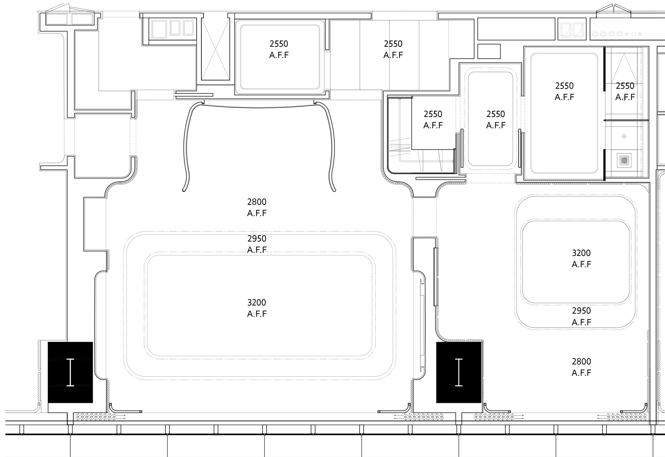
REFLECTED CEILING PLAN 天花平面图
