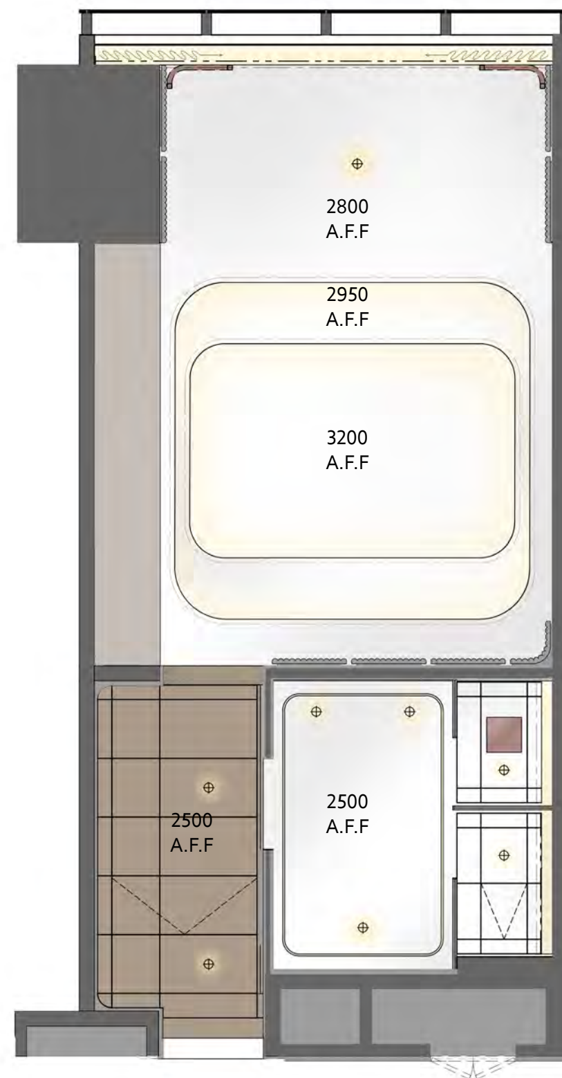
OPTION 2 - TYPE A RCP 方案二 - A型客房天花图
