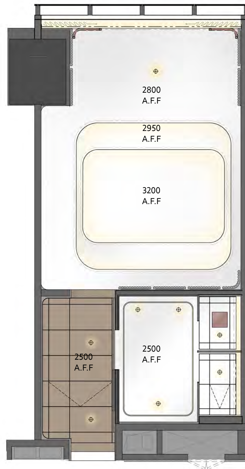
OPTION 1 - TYPE A RCP 方案一 - A型客房天花图
