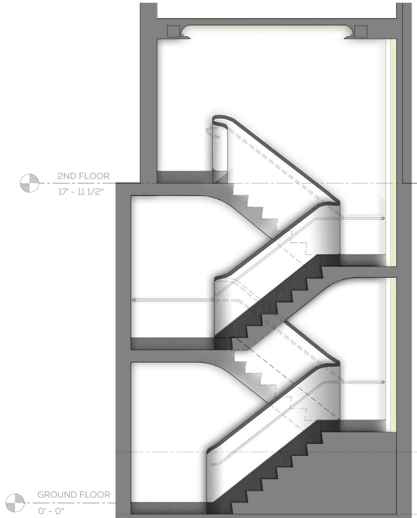
5 STAIR CASE SECTION N.T.S.
