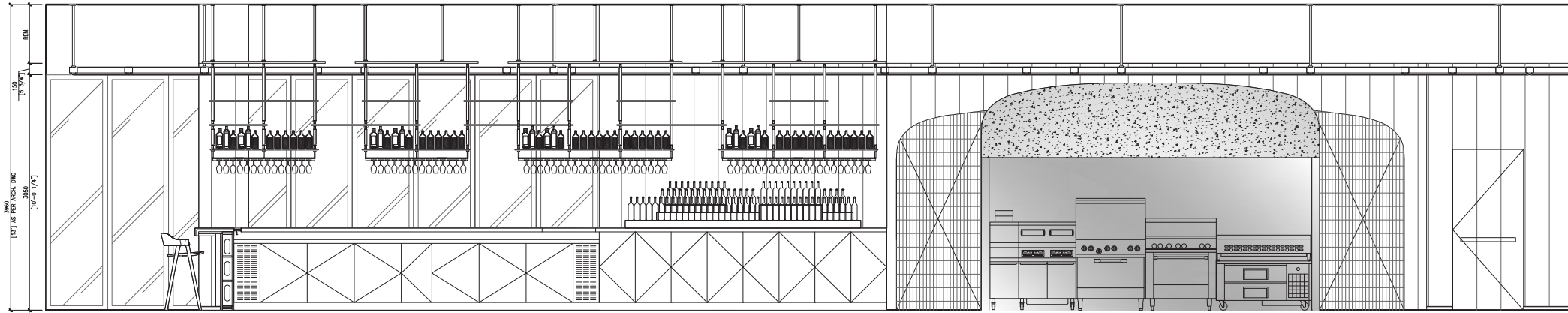
7 ELEVATION N.T.S
