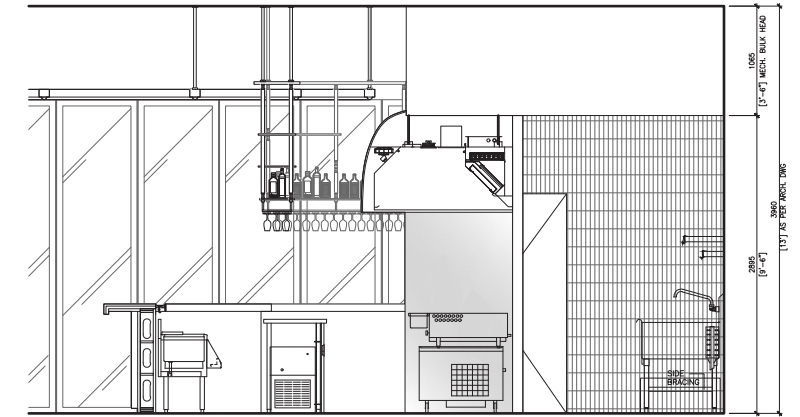
6 ELEVATION N.T.S
