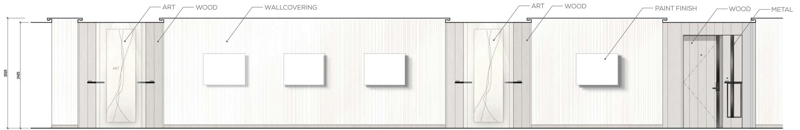
ELEVATION
