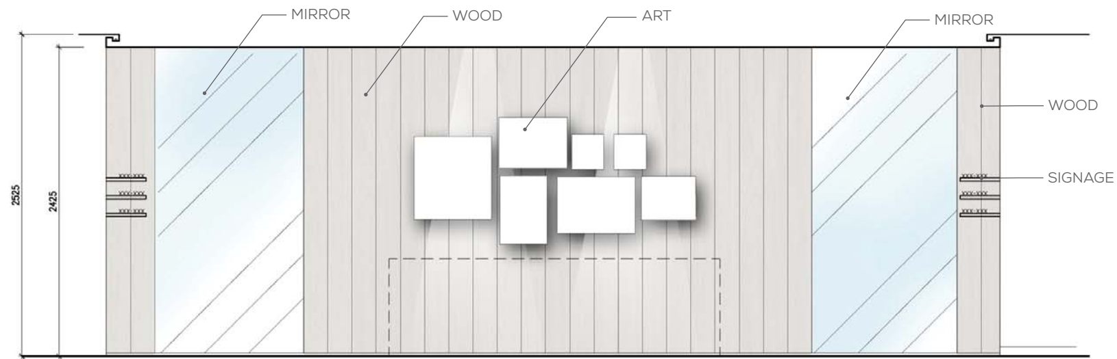
ELEVATION A
