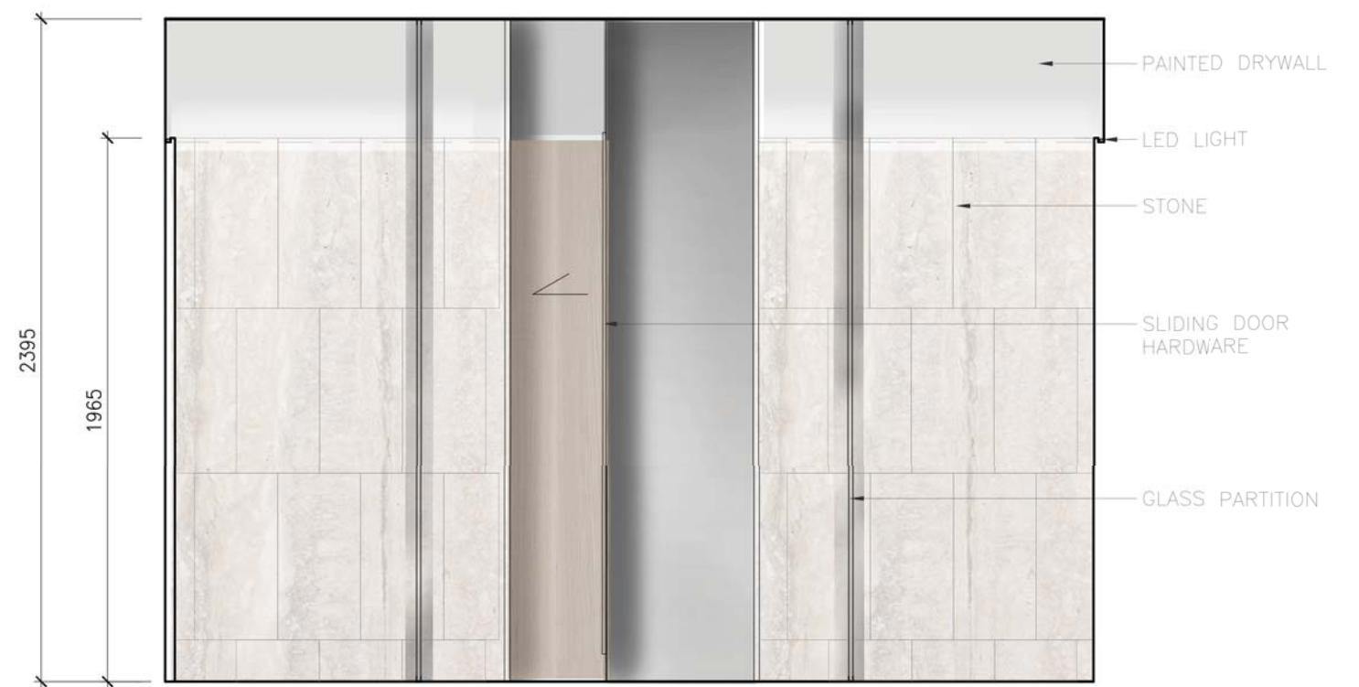
ELEVATION 6
