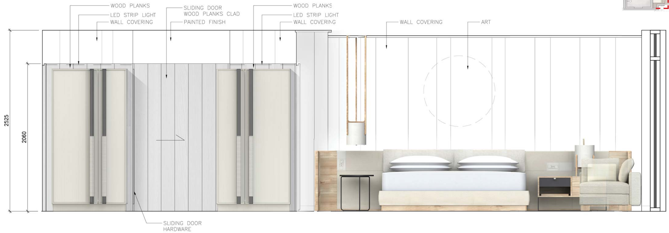
ELEVATION 1
