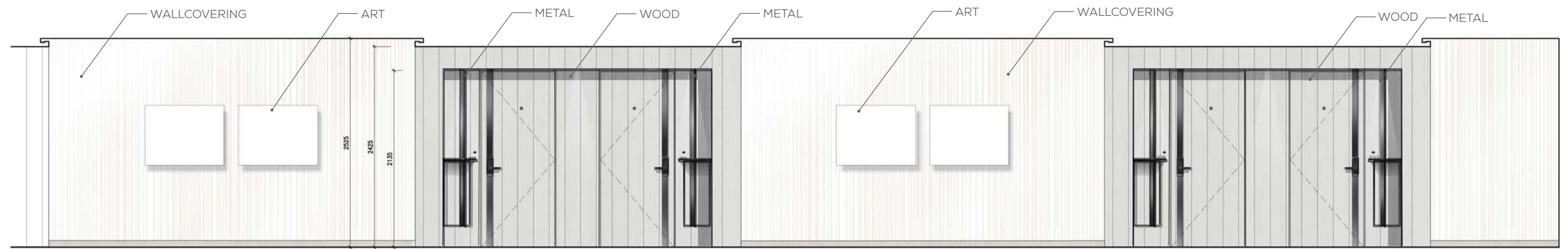
ELEVATION
