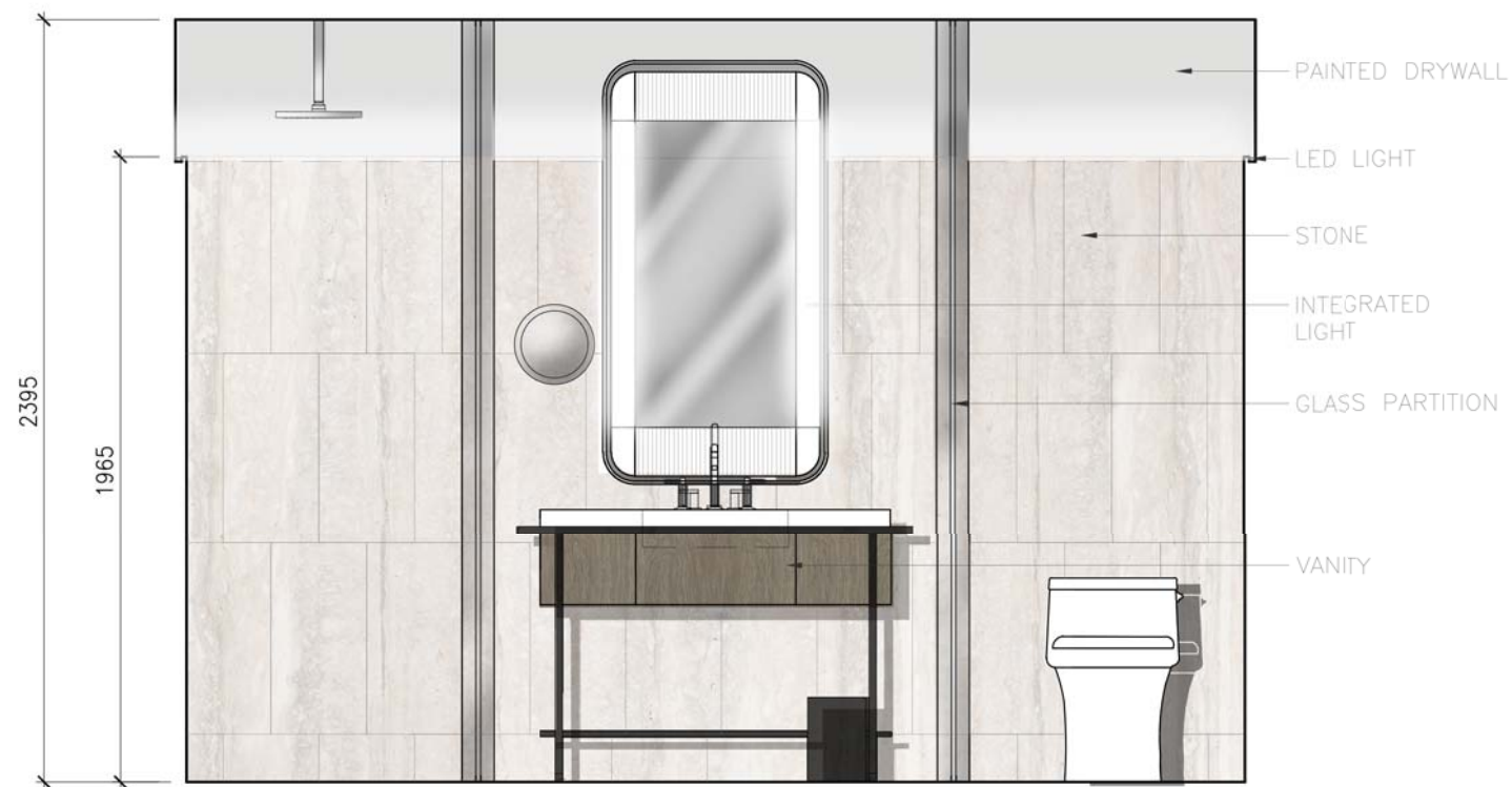
ELEVATION 5
