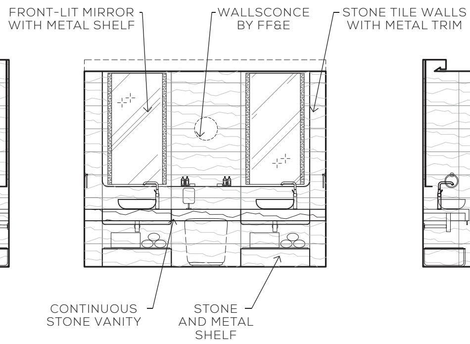
2 ELEVATION
