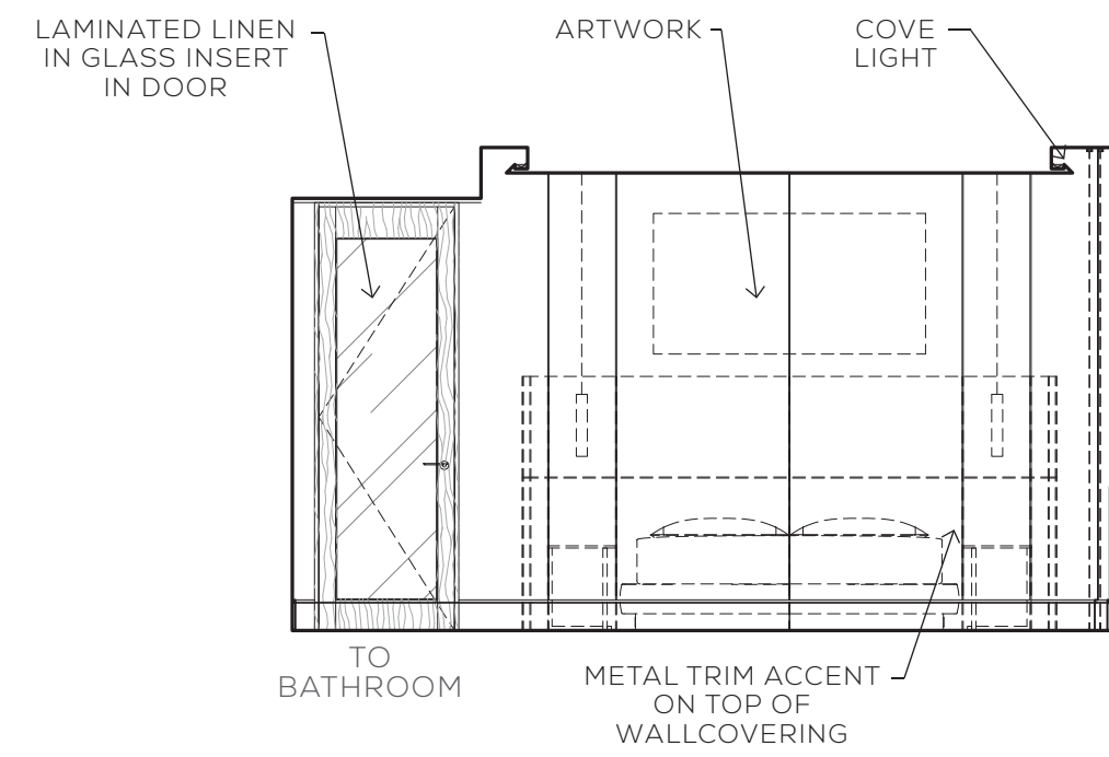
3 ELEVATION
