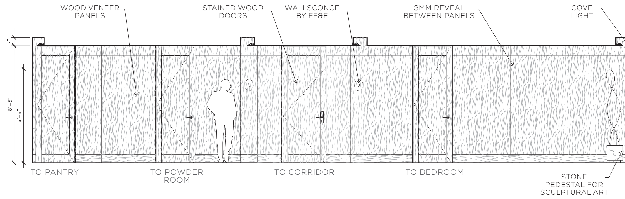
1 ELEVATION
