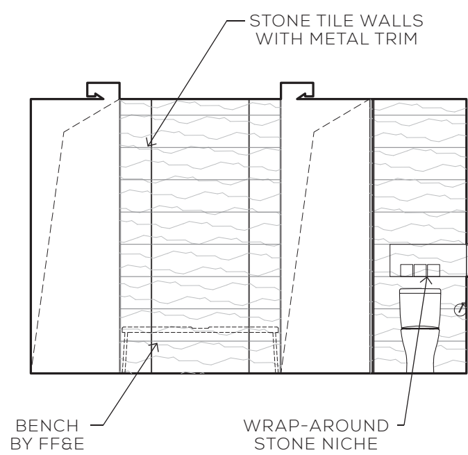
6 ELEVATION
