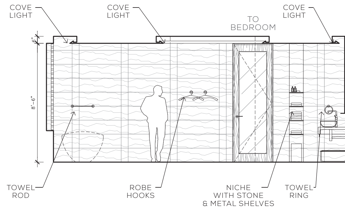
1 ELEVATION
