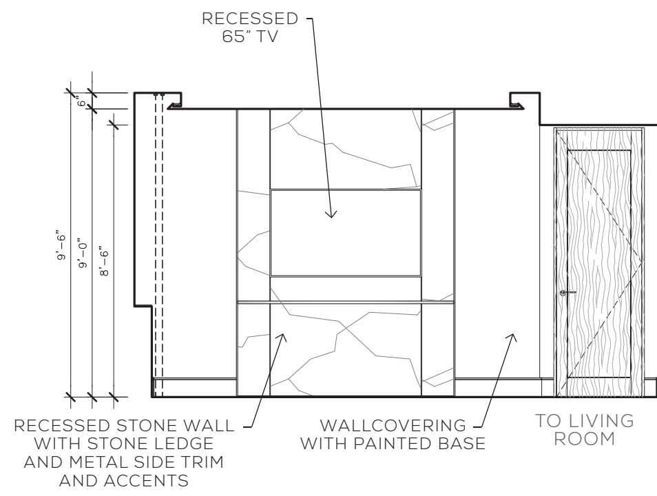
1 ELEVATION
