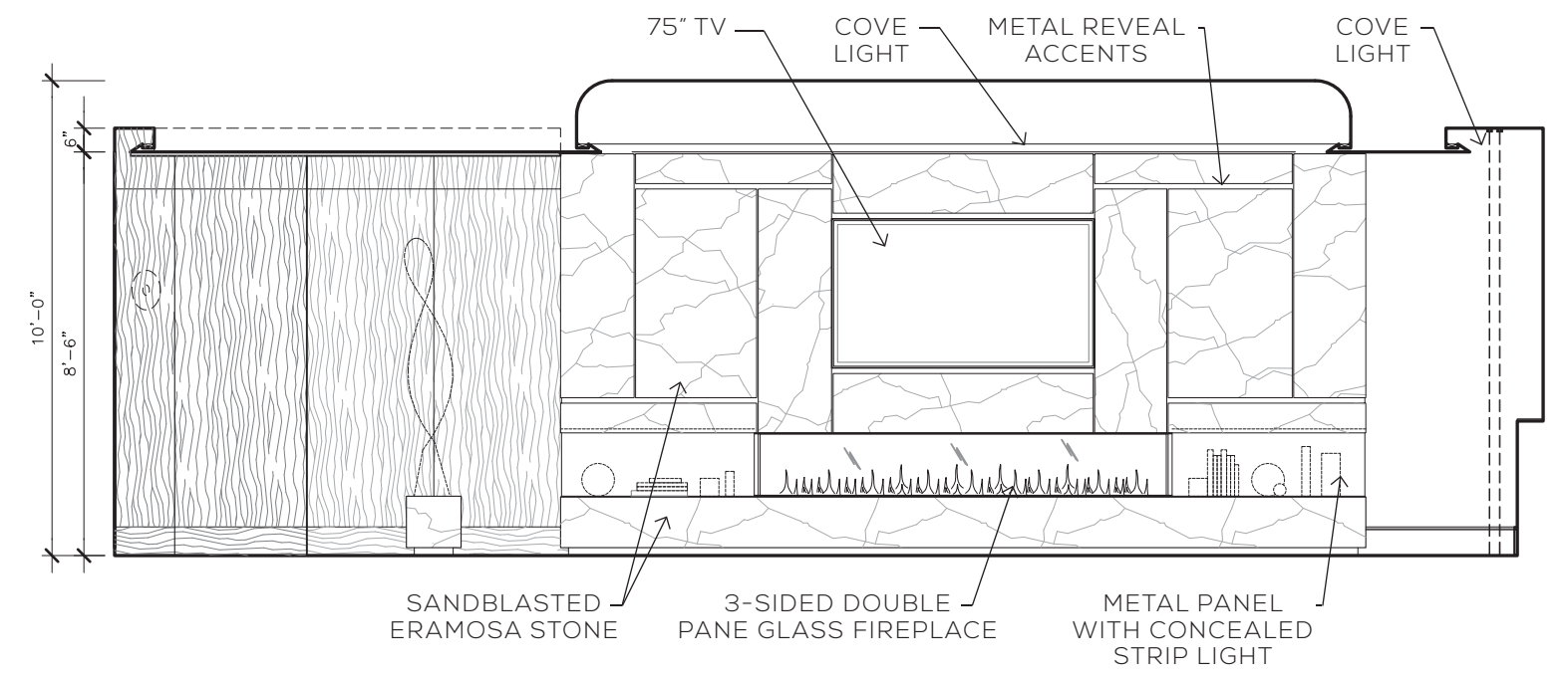
2 ELEVATION
