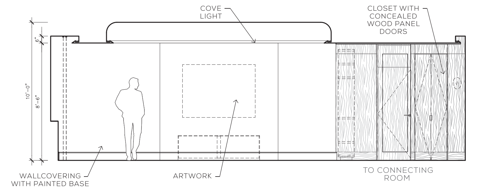
4 ELEVATION
