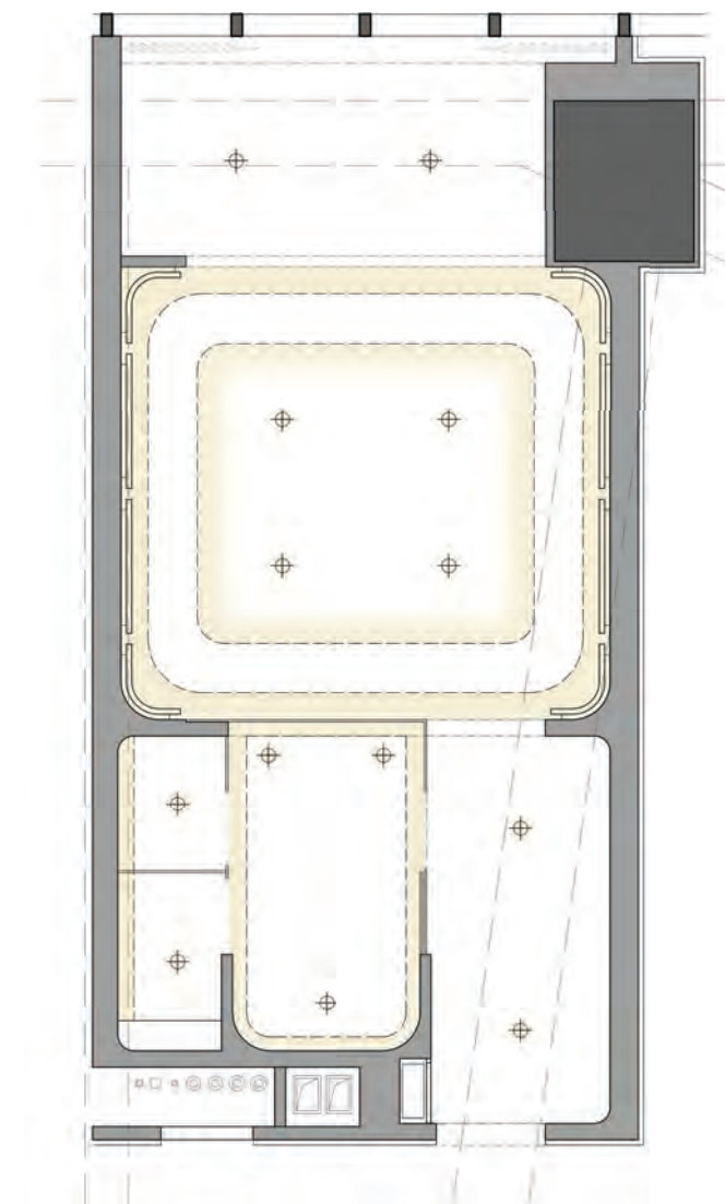
GUESTROOM TYPE A (MUR DOUBLE QUEEN) 标准客房A型 (样板双床房) DOUBLE QUEEN BEDROOM - RCP 双床房 - 天花反向图
